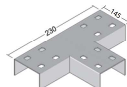
Caixa derivação "C" 38x76 "C" Junction box for double channel
