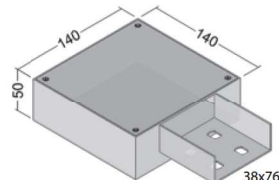
Cx. derivação "L" esquerda 38x76 - 38x38 "L" Left junction box for channel
