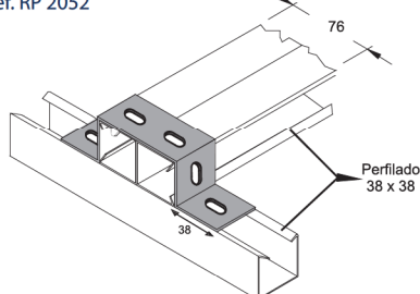
Distanciador "U" triplo Triple "U" distance piece
